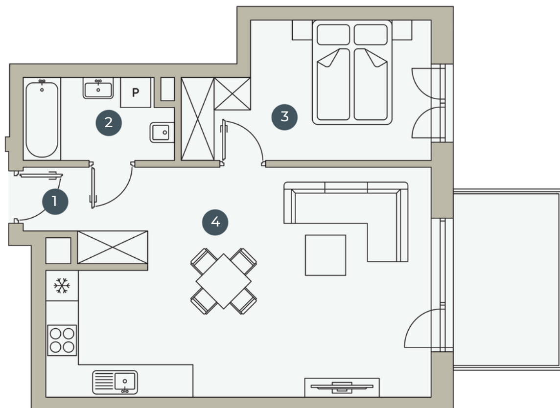
BUDYNEK 48a PIĘTRO 1
